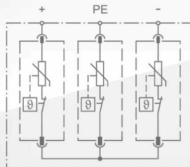
SCHÉMA ZAPOJENÍ
