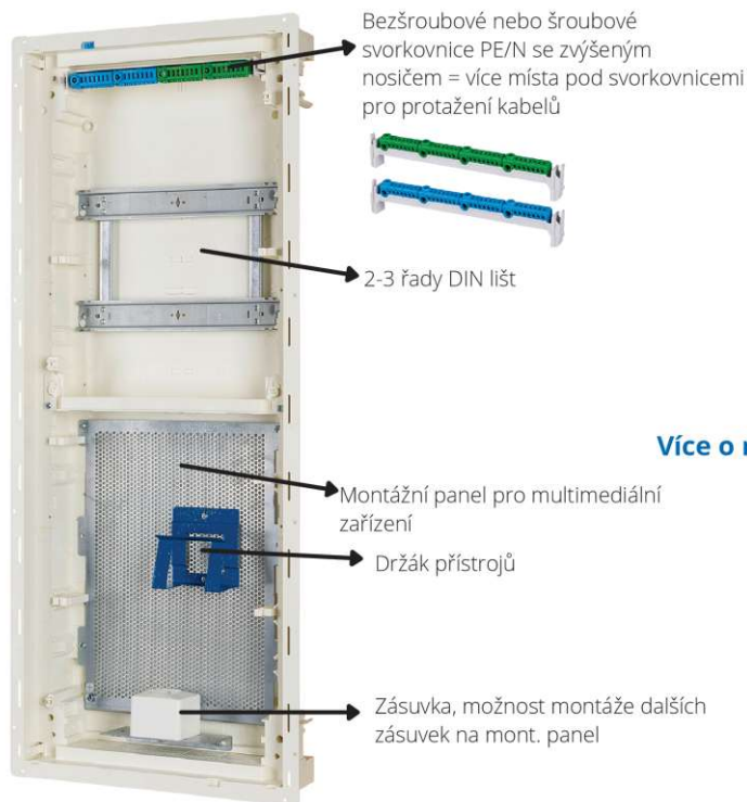
Obr. 3 Rozvodnice KLV v hybridním provedení
