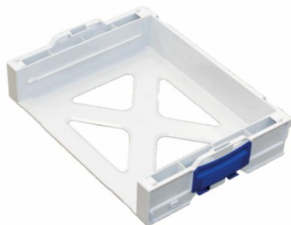
do přihrádky PLBOXXRA lze vložit organizér PIBOXX72H3 a šuplík PLBOXXESF72... k tomu slouží boční vodící lišta
